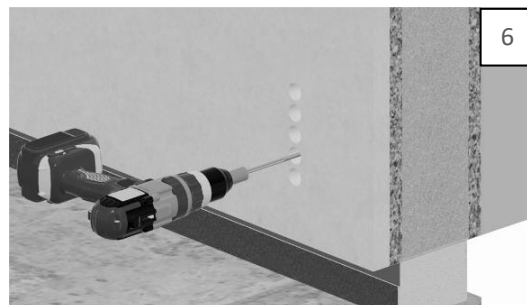
Plaats de wand en verbind deze met het ISP hold down anker d.m.v. de meegeleverde schroeven
